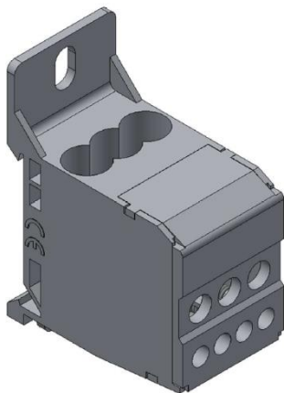
Dimensional Drawing | Plan d'encombrement
